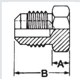
Flare Plug
